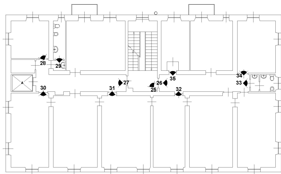
PIANO SECONDO
